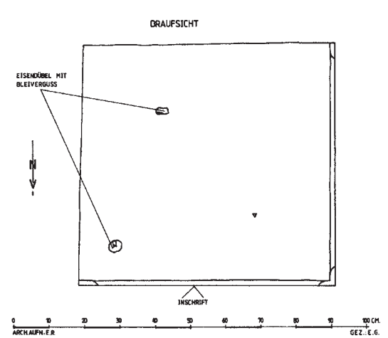
Abb. 30: Statuensockel A42, Oberseite
