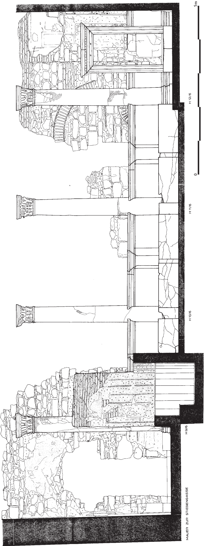
Abb. 24: O-W Schnitt Peristylhof 31a mit Schrankenwand und Brunnen der Südseite
