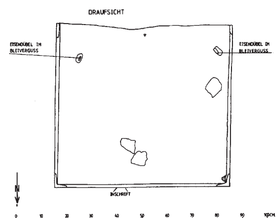
Abb. 35: Statuensockel A43, Oberseite
