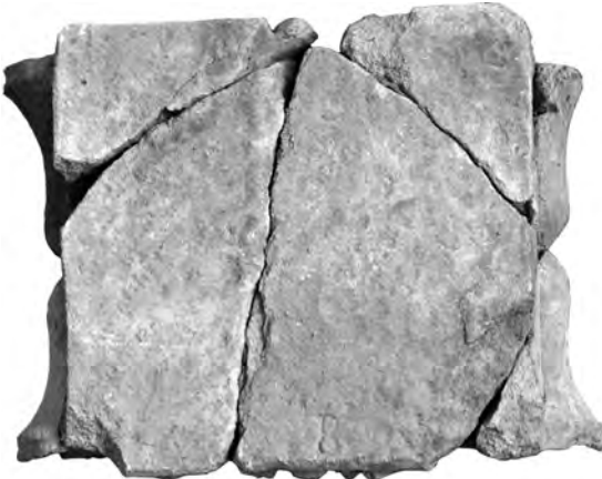
Säulenkaptell A 31b-10, Oberseite
