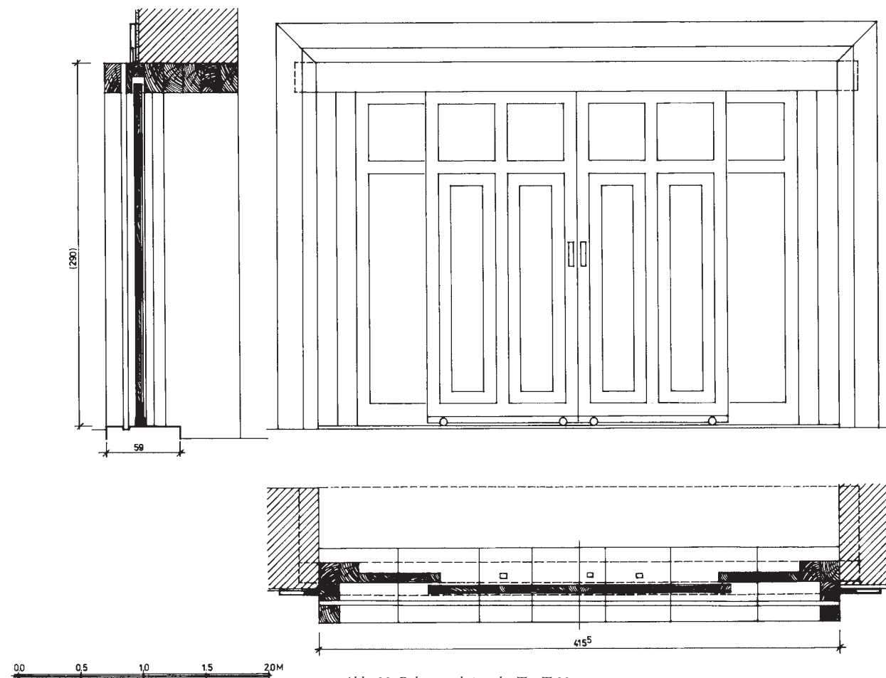
Abb. 33: Rekonstruktion der Tür T 30
