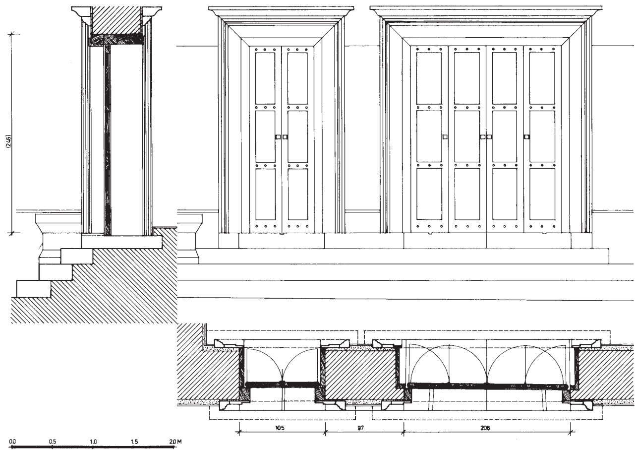
Abb. 46: Rekonstruktion der Türen T 13 und T 14
