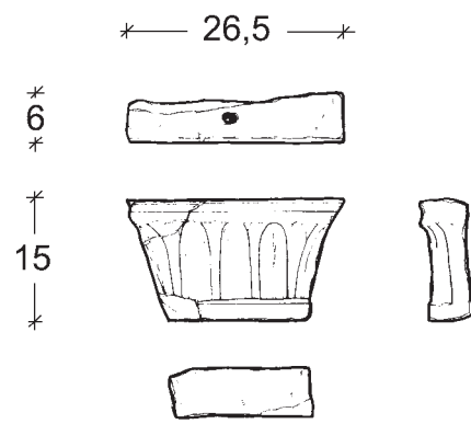
Pilasterkapitell A 31b-11
