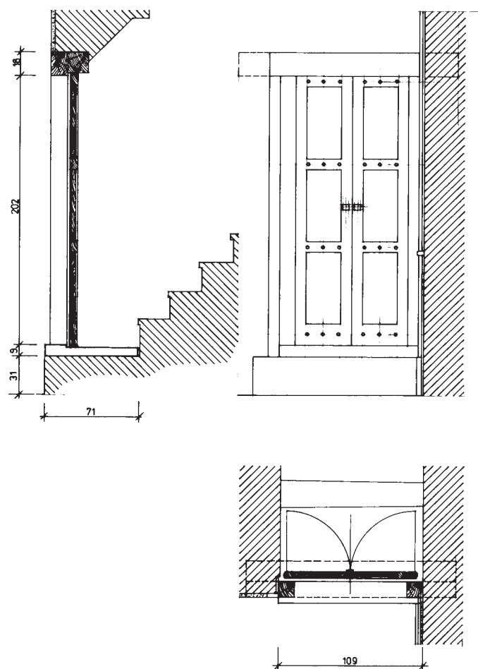
Abb. 54: Rekonstruktion der Tür T 19
