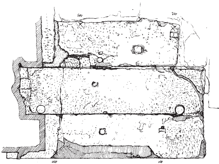
Abb. 21: Tür T 1 mit Türschwelle TS 1 (Eingangsportal an der Alytarchenstoa)
